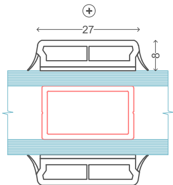
⊖ Standard PVC srosseløsninger Limt på begge sider 27 mm + Duplex på innsiden 2-lag glass
