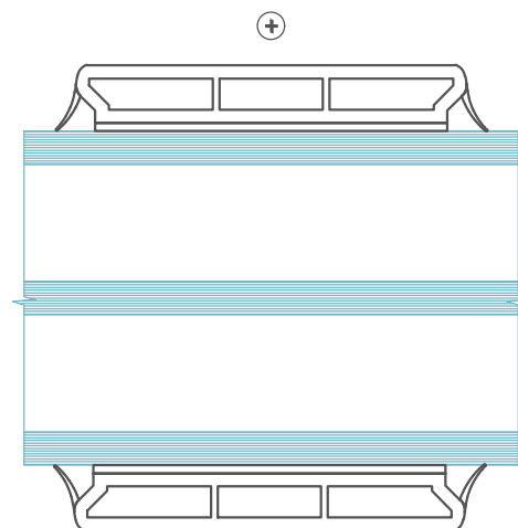
⊖ Standard PVC sprosseløsninger Limt på begge sider 47 mm 3-lag glass
