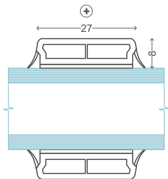
⊖ Standard PVC sprosseløsninger Limt på begge sider 27 mm 2-lag glass
