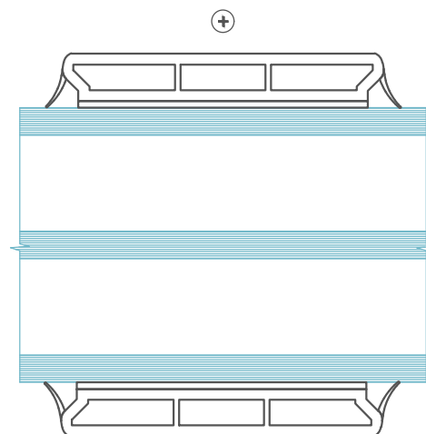
⊖ Standard PVC sprosse Limet på begge sider 47mm 3-lags isolerede ruder
