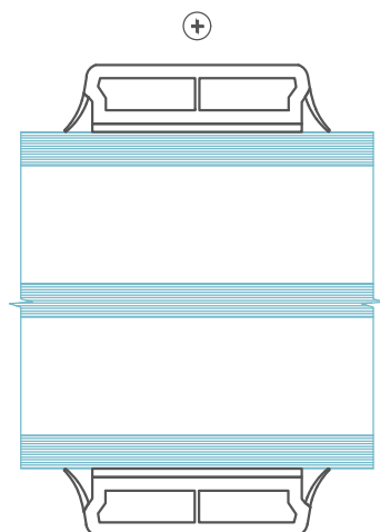
⊖ Standard PVC sprosse Limet på begge sider 27mm 3-lags isolerede ruder
