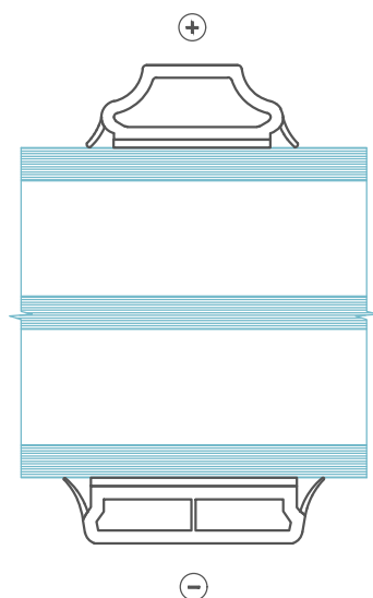
Kombinert PVC sprosseløsninger Limt på begge sider: Standard 27mm på utsiden Klassiske 22mm på innsiden 3-lag glass
