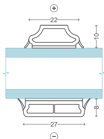
Kombinert PVC sprosseløsninger Limt på begge sider: Standard 27mm på utsiden Klassiske 22mm på innsiden 2-lag glass
