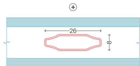
⊖ Sprosseløsninger inne i glasset 26 mm 2-lag glass
