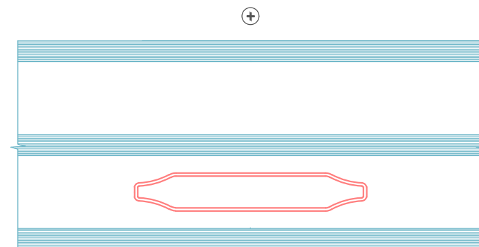
⊖ Sprosseløsninger inne i glasset 45 mm 3-lag glass
