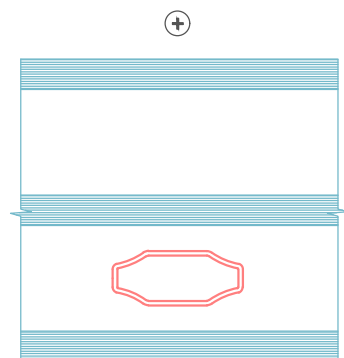
⊖ Sprosseløsninger inne i glasset 18 mm 3-lag glass
