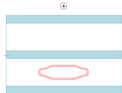
⊖ Sprosseløsninger inne i glasset 26 mm 3-lag glass
