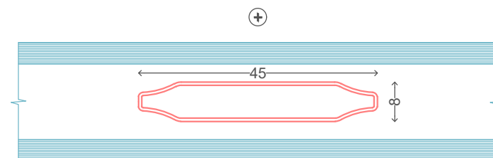
⊖ Sprosseløsninger inne i glasset 45 mm 2-lag glass
