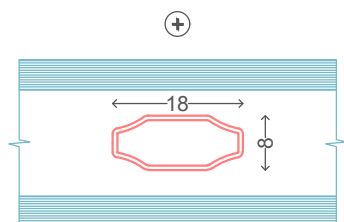
⊖ Sprosseløsninger inne i glasset 18 mm 2-lag glass
