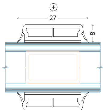
⊖ Standard PVC sprosseløsninger Limt på begge sider 27mm + Duplex på innsiden 2-lags glass
