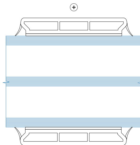
⊖ Standard PVC sprosse Limet på begge sider 47mm 3 -lags isolerede ruder
