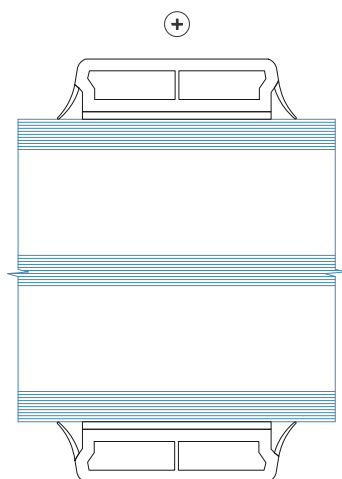
⊖ Standard PVC srosseløsninger Limt på begge sider 27mm 3-lags glass
