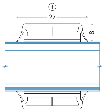
⊖ Standard PVC srosseløsninger Limt på begge sider 27mm 2-lags glass
