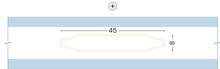
⊖ Sprosseløsninger inne i glasset 45mm 2-lag glass
